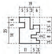
B montante battuta
