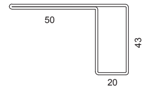
Telaio pressopiegato a richiesta
