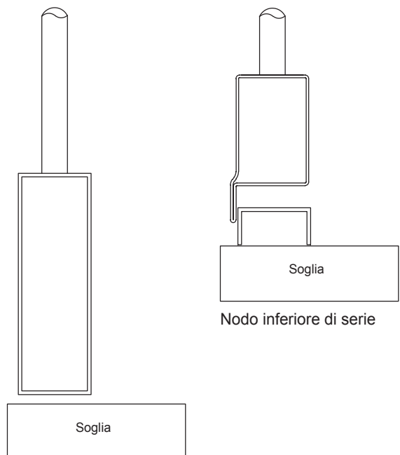
Nodo inferiore a richiesta*
